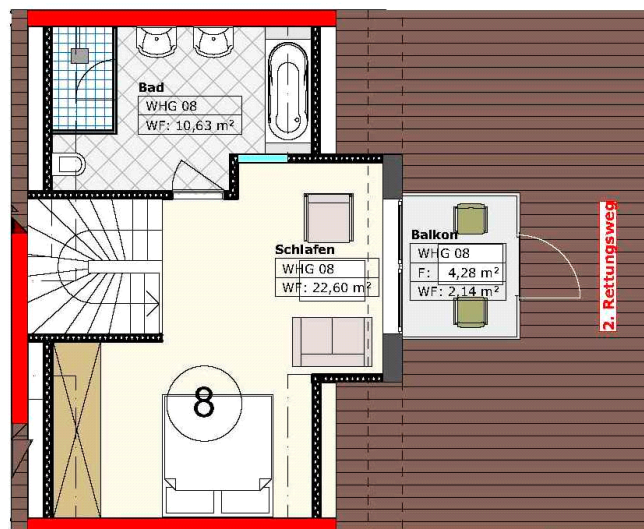
Dachgeschoss
